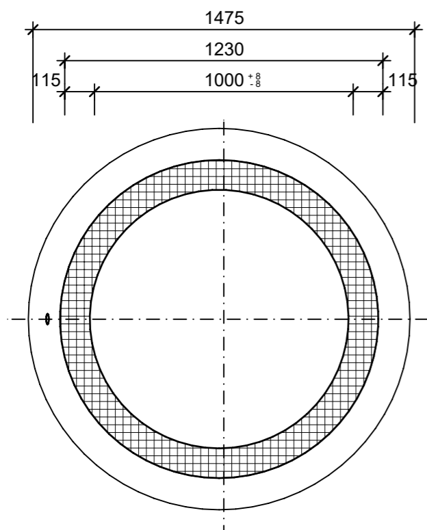
Schnitt 1-1, 1:20
