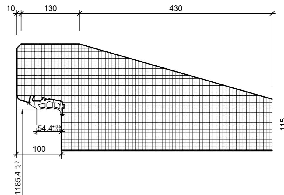
Detail Glockenmuffe, 1:5
