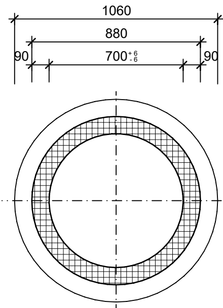
Schnitt 1-1, 1:20
