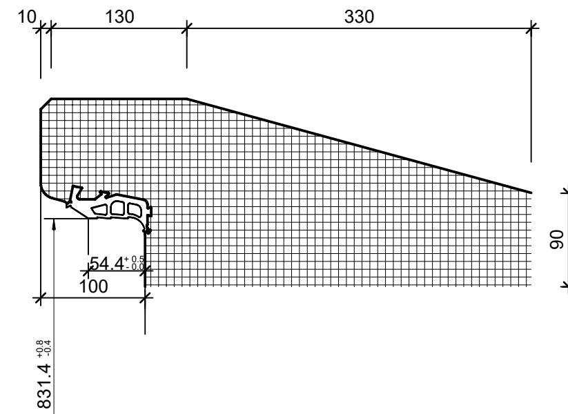
Detail Glockenmuffe, 1:5
