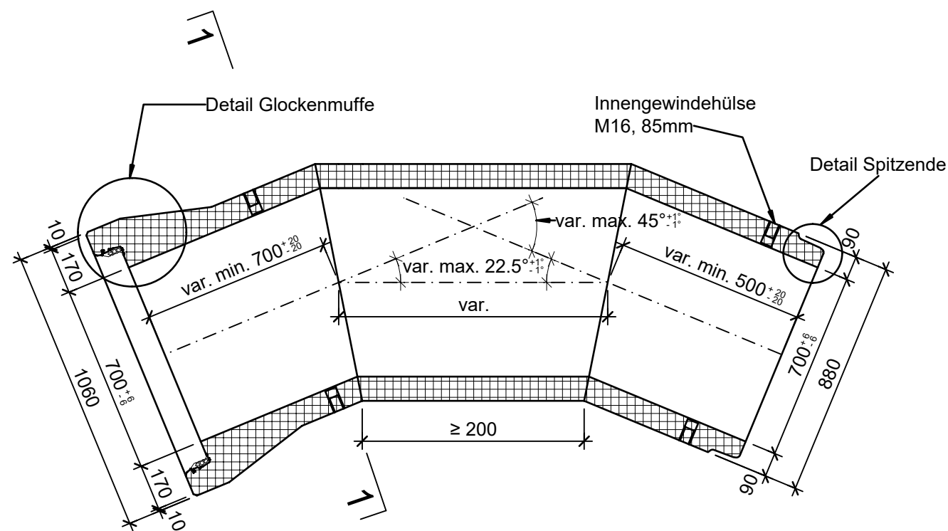
Grundriss, 1:20
