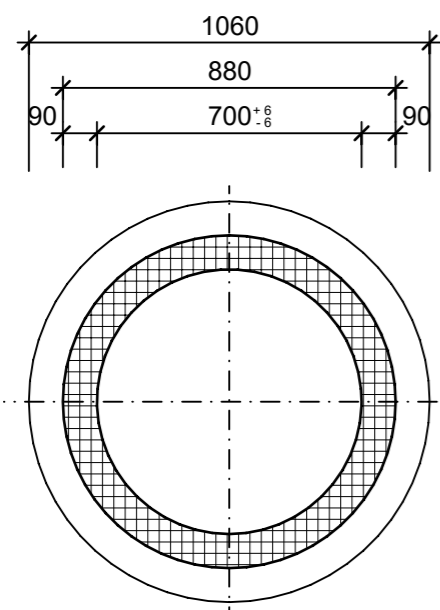
Schnitt 1-1, 1:20
