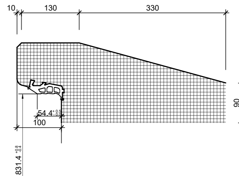
Detail Glockenmuffe, 1:5
