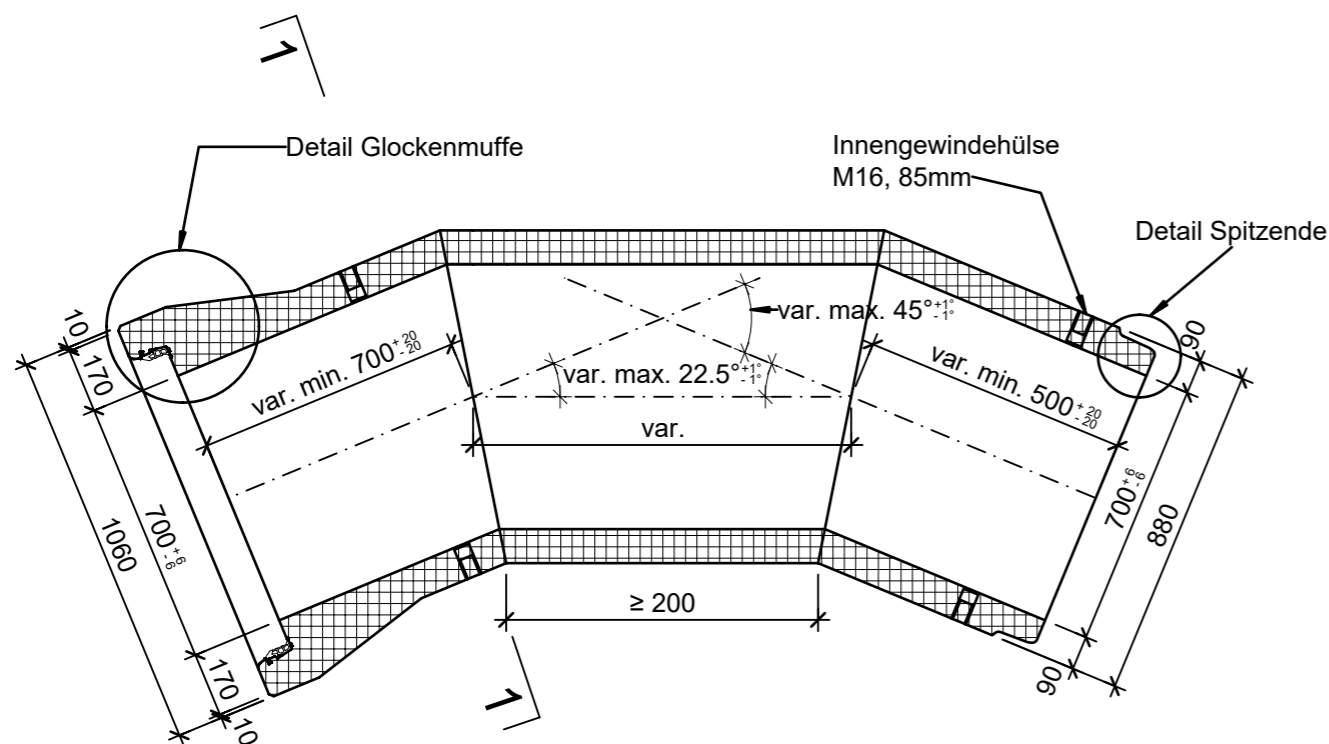
Grundriss, 1:20
