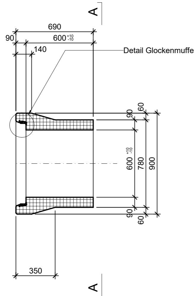
Grundriss, 1:20
