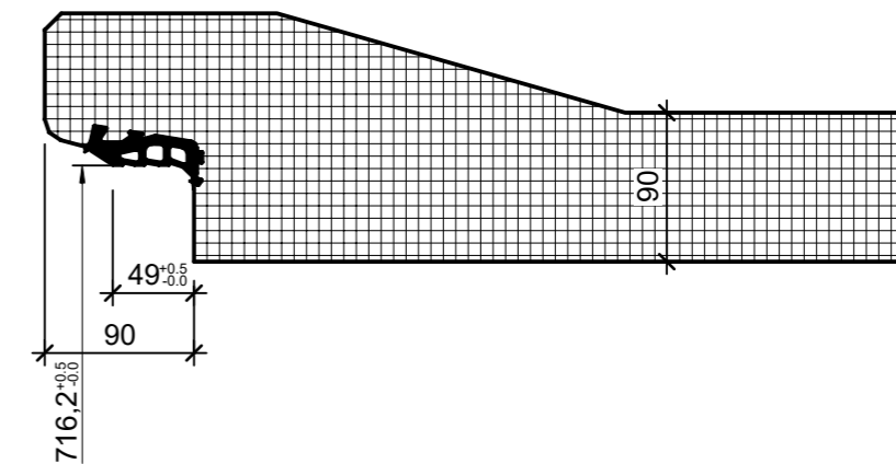
Detail Glockenmuffe, 1:5
