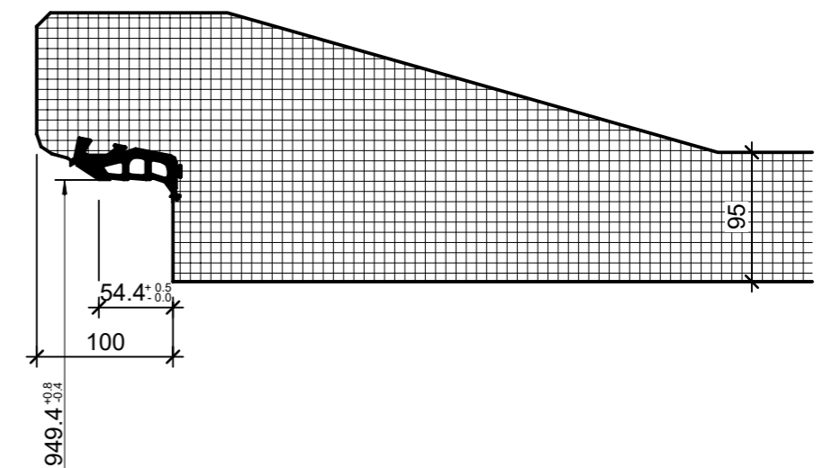
Detail Glockenmuffe, 1:5
