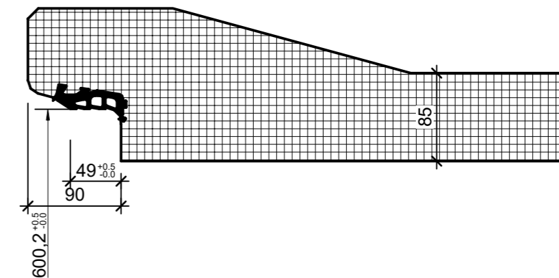
Detail Glockenmuffe, 1:5
