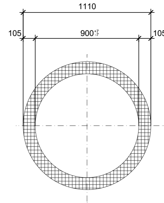
Detail Spitzende, 1:2
