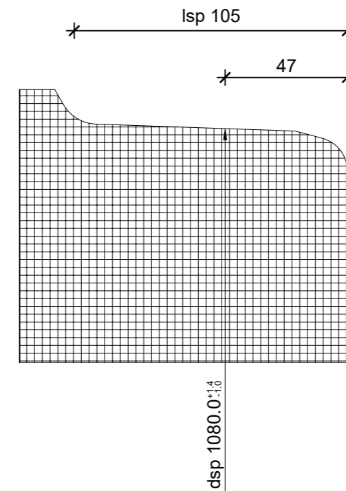
Detail Spitzende, 1:2
