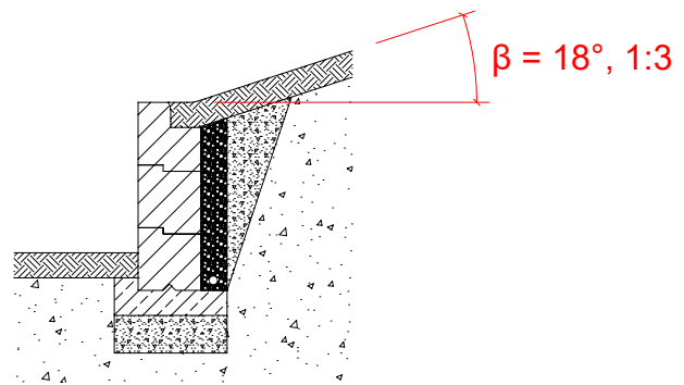
Bild 7 Lastfall D
