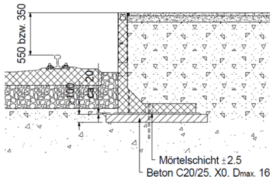
Bild 11: Perronwinkel - Standardprofil
