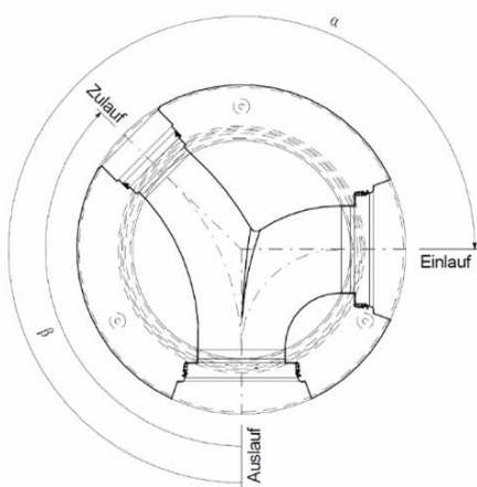
Bild 14: Anschlusswinkel bei CENTUB® Massschachtunterteilen
