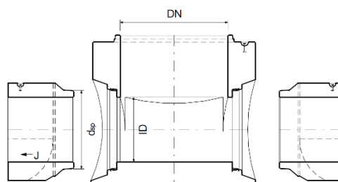
Bild 4: Anschluss mit MAROWA Röser Hochleistungsbetonrohren mit Gefälle J ≤ 150 ‰
