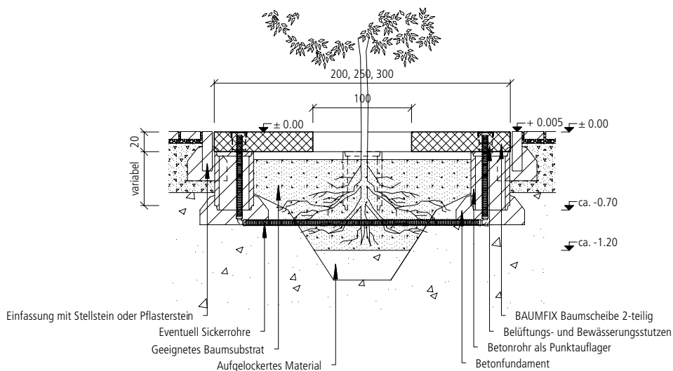
Einbauschema BAUMFIX® Baumscheiben auf Punktaulager (z. B. Betonrohre DN 300)
