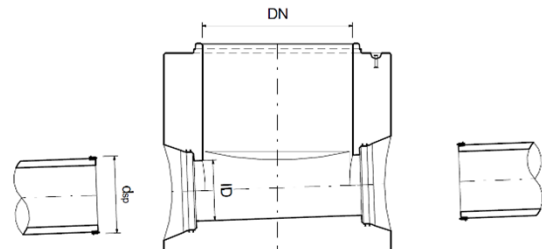
Bild 6: Anschluss mit Steinzeugrohre Typ H mit Gefälle J ≤ 150 ‰
