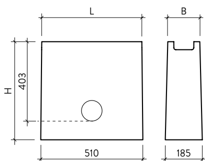
Bild 4: Liniensinkkasten Typ 1
