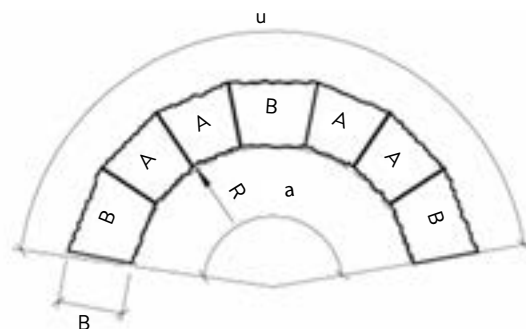
Bild 31: Optimale Muffenbildung
