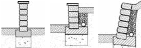
Freistehende Mauer Stützmauer Stützmauer mit Anzug Bild 4: Mögliche Anwendungen der SANTURO® Mauersteine
