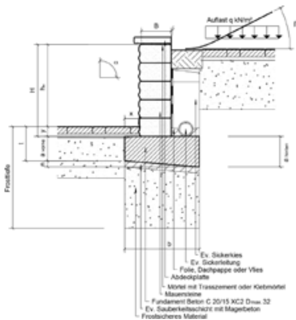
Bild 40: Aufbauquerschnitt
