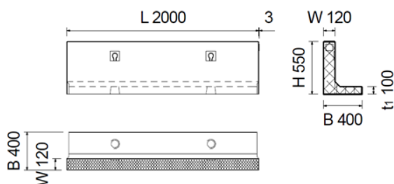
Bild 7: Perronwinkel Typ 7
