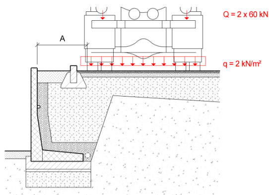
Bild 13: Lastfall C4
