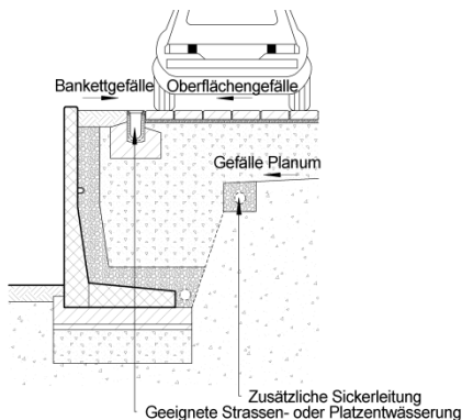
Bild 23: Zusätzliche Entwässerung
