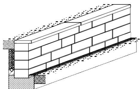
Bild 26: Stützmauer
