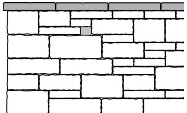
Mauertyp 20, Mauerhöhe 0.98 m
