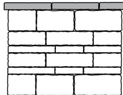
Mauertyp 15, Mauerhöhe 0.90 m
