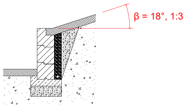
Bild 7 Lastfall D
