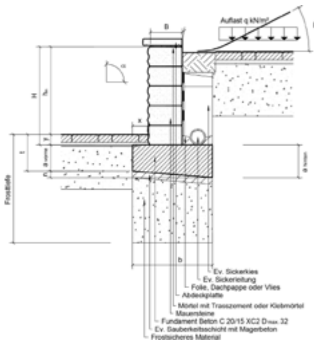
Bild 46: Vertikaler Maueraufbau
