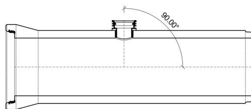
Bild 4: Anschlusswinkel DENSO Steckanschlusstück
