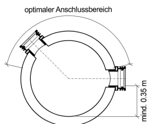
Bild 3: Anschlussmöglichkeiten DENSO Steckanschlusstück
