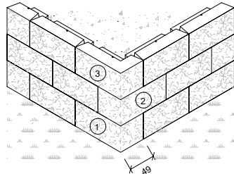
Bild 13 FELSMAUER Böschungselemente – Schematische Darstellung einer Aussenecke (① Anfangseckstein rechts; ② Mitteleckstein links, ③ Schlus-eckstein rechts)
