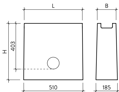
Bild 4: Liniensenkkasten Typ 1
