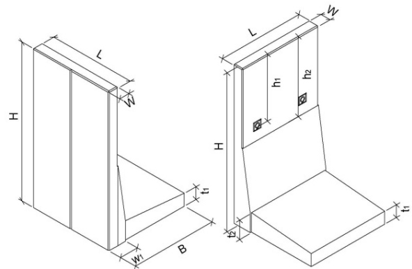
Bild 6: EXACTA® Winkelplatte Typ 2
