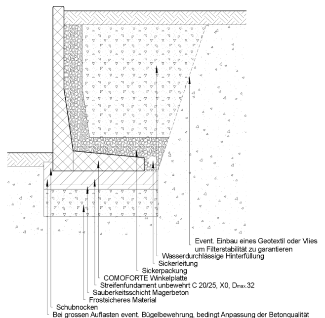
Bild 19: Schematische Darstellung des Aufbaus mit Streifenfundament
