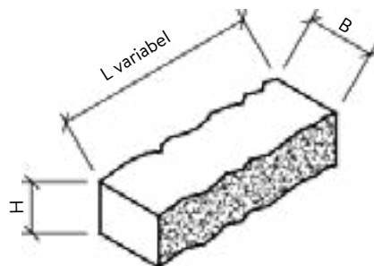
Bild 10: Technische Zeichnung SANTURO® Spaltmauerstein 2seitig gespalten
