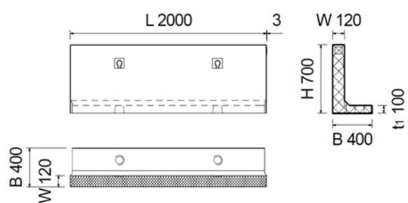
Bild 6: Perronwinkel Typ 6
