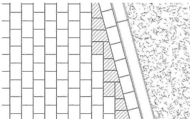
Bild 29: Mögliches Verlegebild beim Anschluss von schräg verlaufende Abschlusssänder, schraffierte Steine zeigen die zugeschnittenen Passsteine
