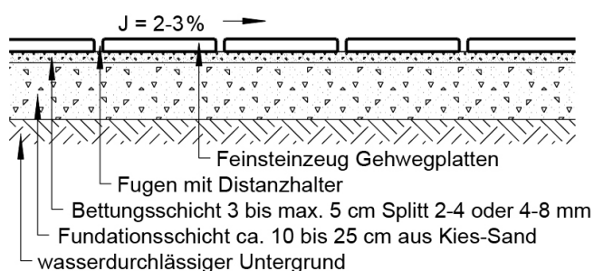
Bild 3: Aufbau des Plattenbelages über einer Foundationsschicht
