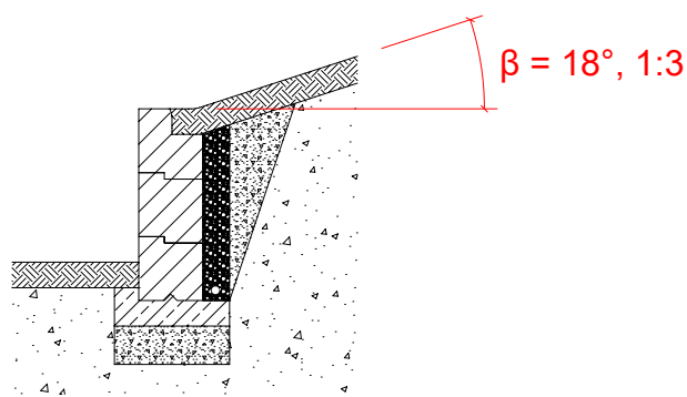
Bild 7 Lastfall D
