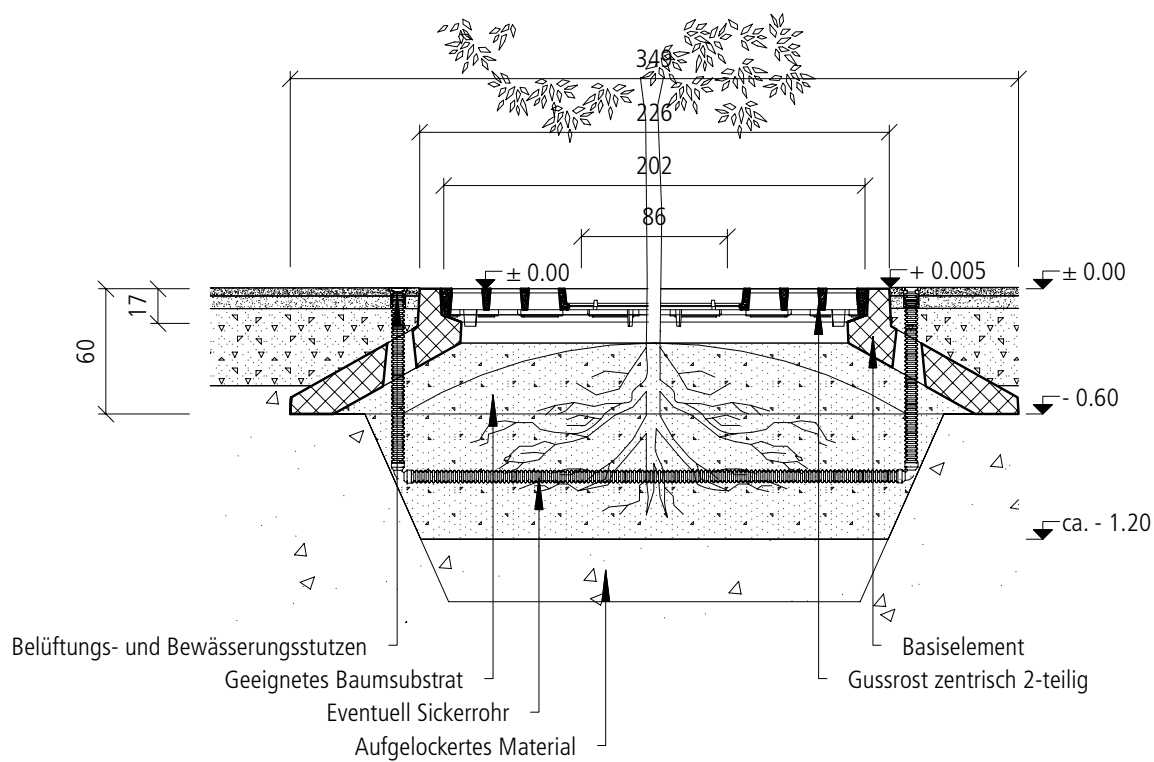
Einbauschema COPAL® CUPOLA Baumwurzelschutz mit Gussrost
