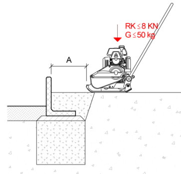
Bild 10: Lastfall F
