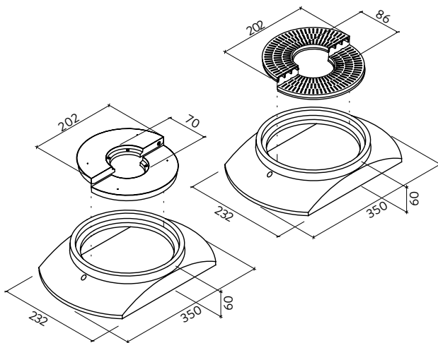
Kombinationsmöglichkeiten COPAL® CUPOLA Baumwurzelraumschutz
