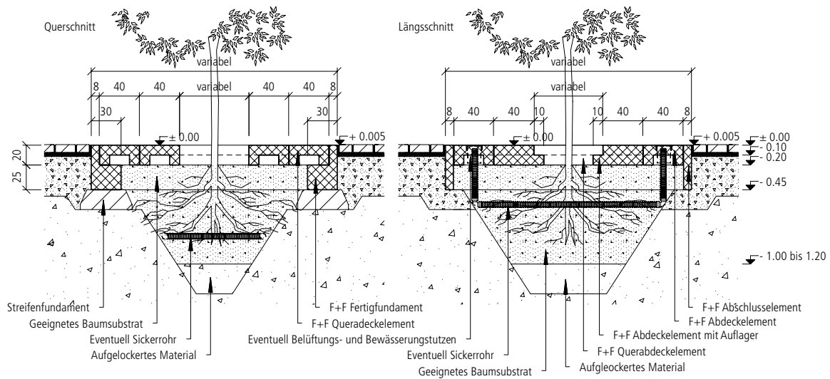
Einbauschema F+F Baumwurzelraumschutz mit Fertigteilfundamenten und Abschlusselementen
