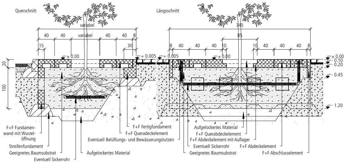
Einbauschema F+F Baumwurzelraumschutz mit Fundamentwand mit Wurzelöffnungen, Fertigteilfundament und Abschlusselement
