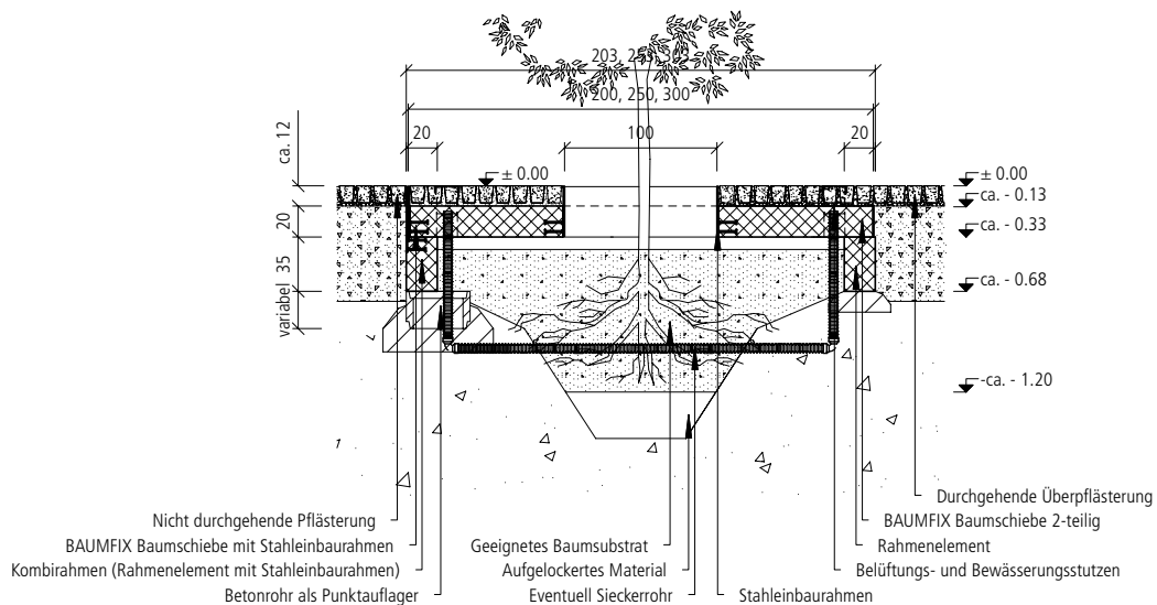
Einbauschema BAUMFIX® Baumscheiben mit Rahmenelement und Überpflasterung (Variante Unterflur)
