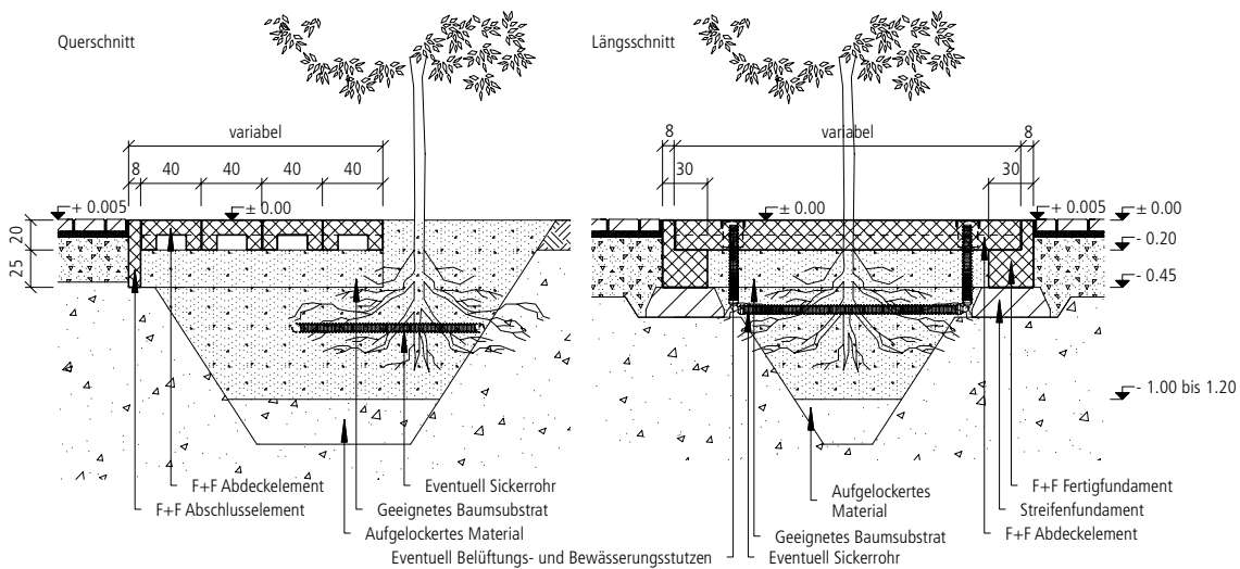
Einbauschema F+F Baumwurzelraumschutz als Wegbrücke mit Fertigteilfundament und einem Abschlusselement
