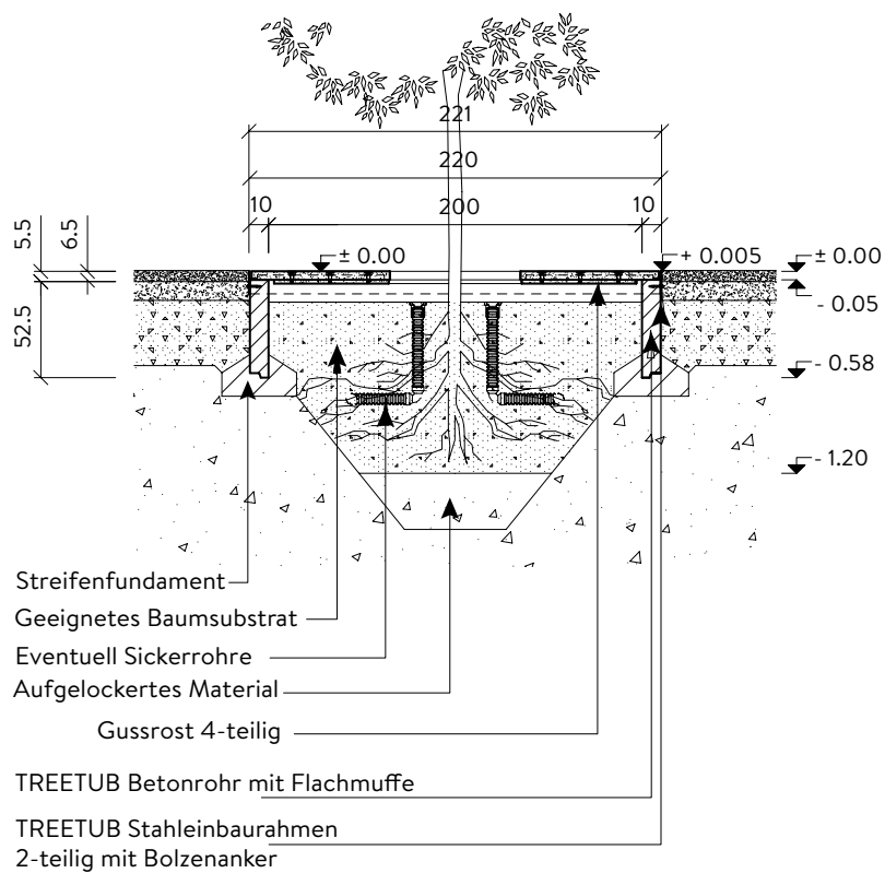
Einbauschema TREETUB Baumwurzelraumschutz mit Gussrost
