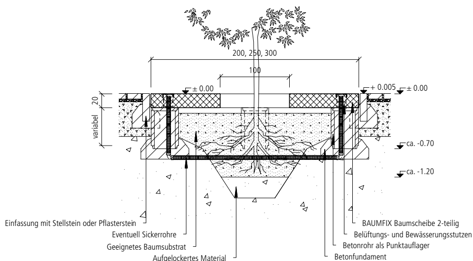
Einbauschema BAUMFIX® Baumscheiben auf Punktaflager (z. B. Betonrohre DN 300)
