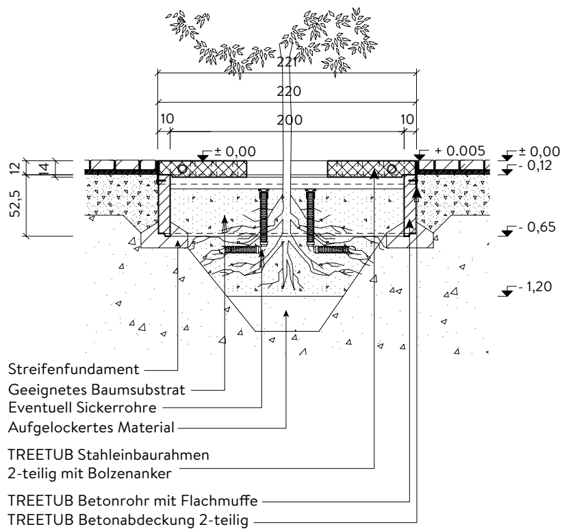
Einbauschema TREETUB Baumwurzelraumschutz mit Betonabdeckung
