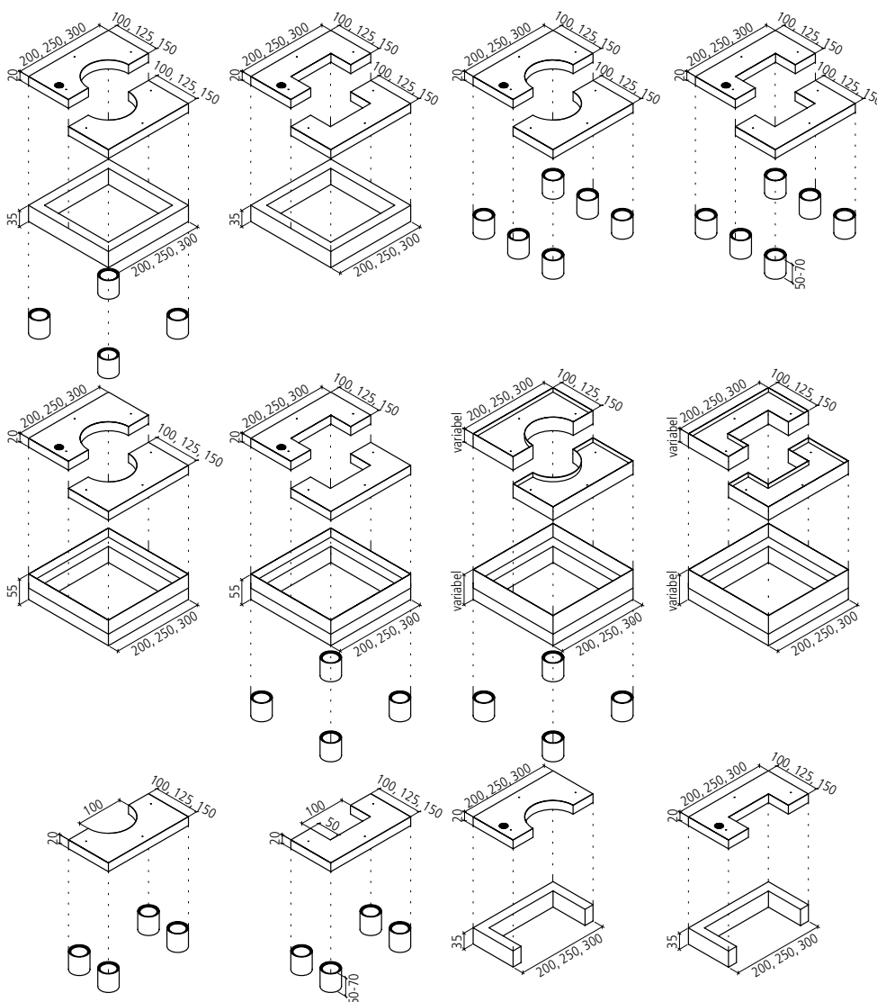
Kombinationsmöglichkeiten BAUMFIX® Baumscheiben
