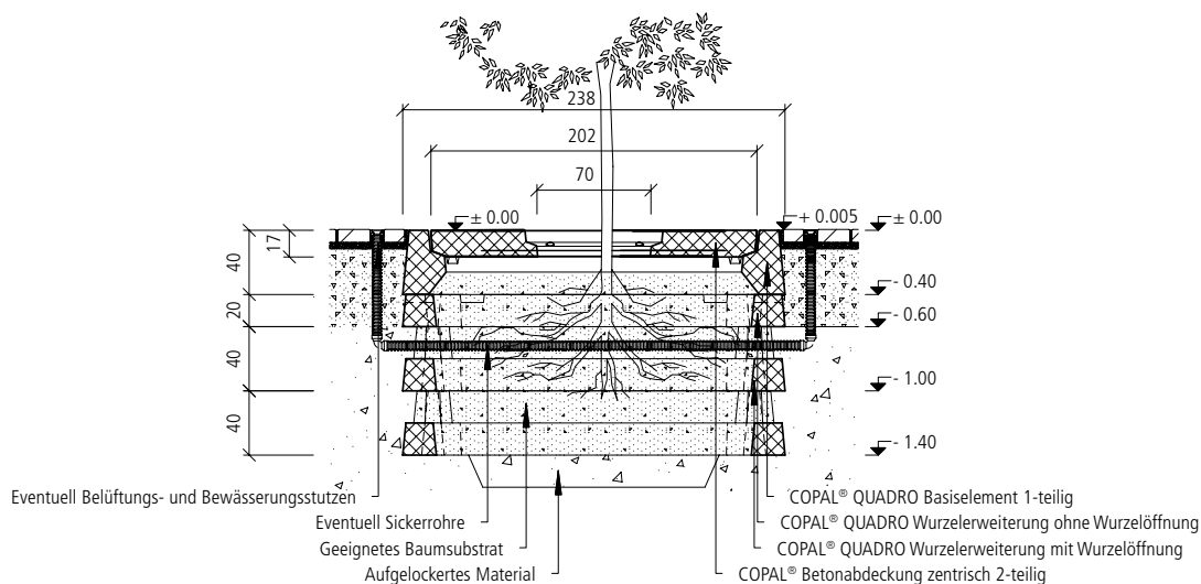
Einbauschema COPAL® QUADRO Baumwurzelraumschutz mit Betonabdeckung exzentrisch und Wurzelraumerweiterung mit Wurzelöffnungen
