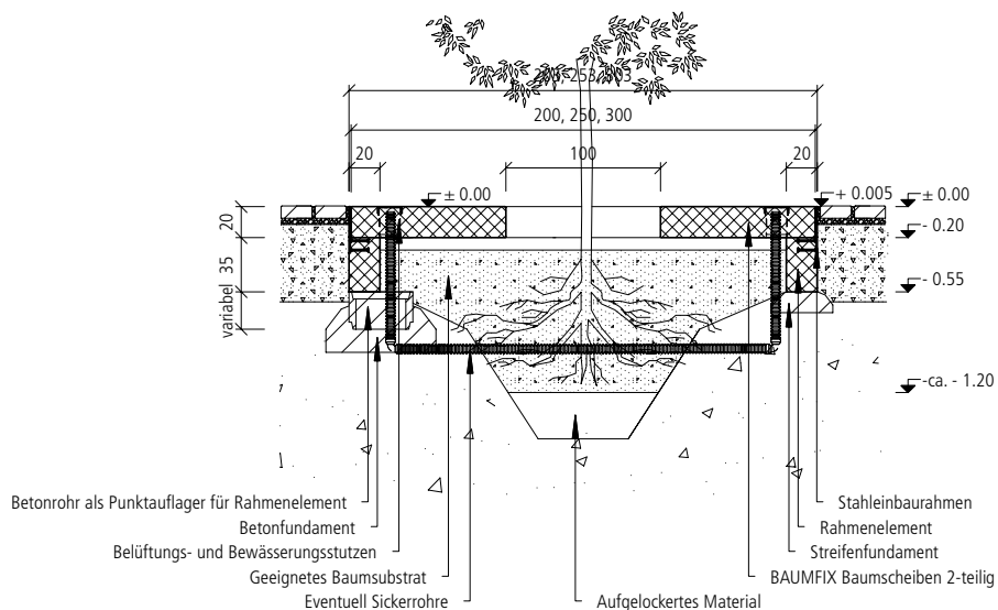
Einbauschema BAUMFIX® Baumscheiben mit Rahmenelement
