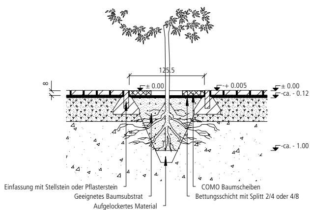
Einbauschema COMO Baumscheiben ohne Fundamentrahmen
