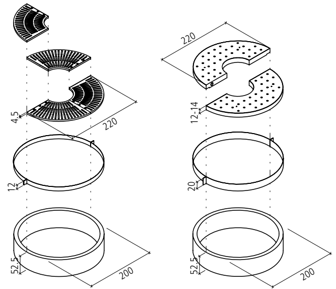
Kombinationsmöglichkeiten TREETUB Baumwurzelraumschutz
