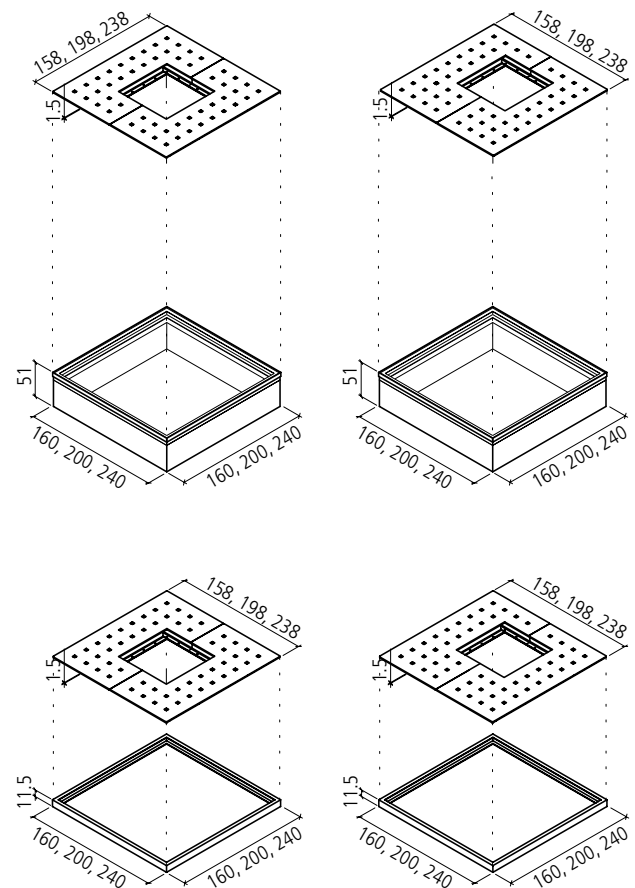
Kombinationsmöglichkeiten COPAL® STEEL Stahlbaumscheibe
