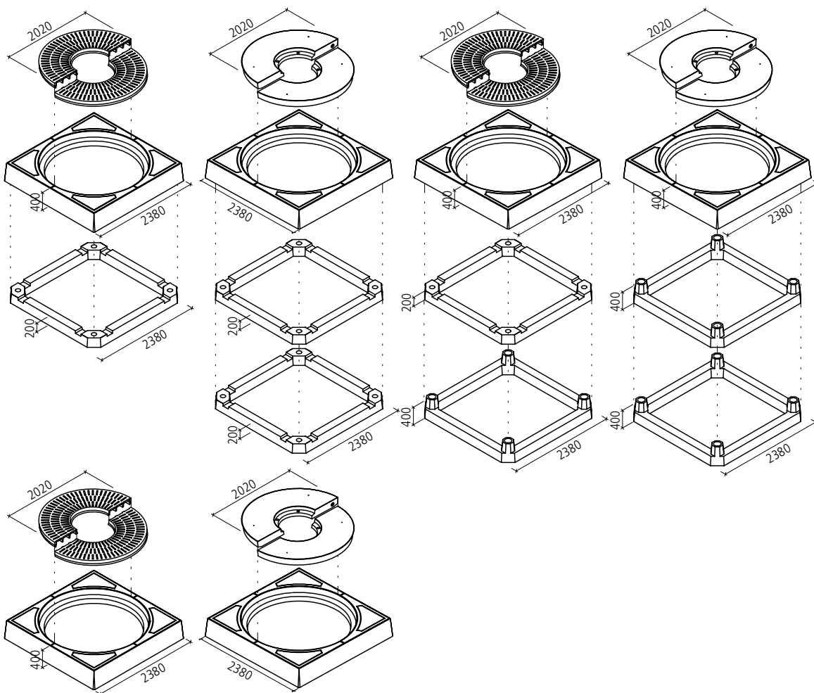
Versetzen der COPAL® Betonabdeckung
